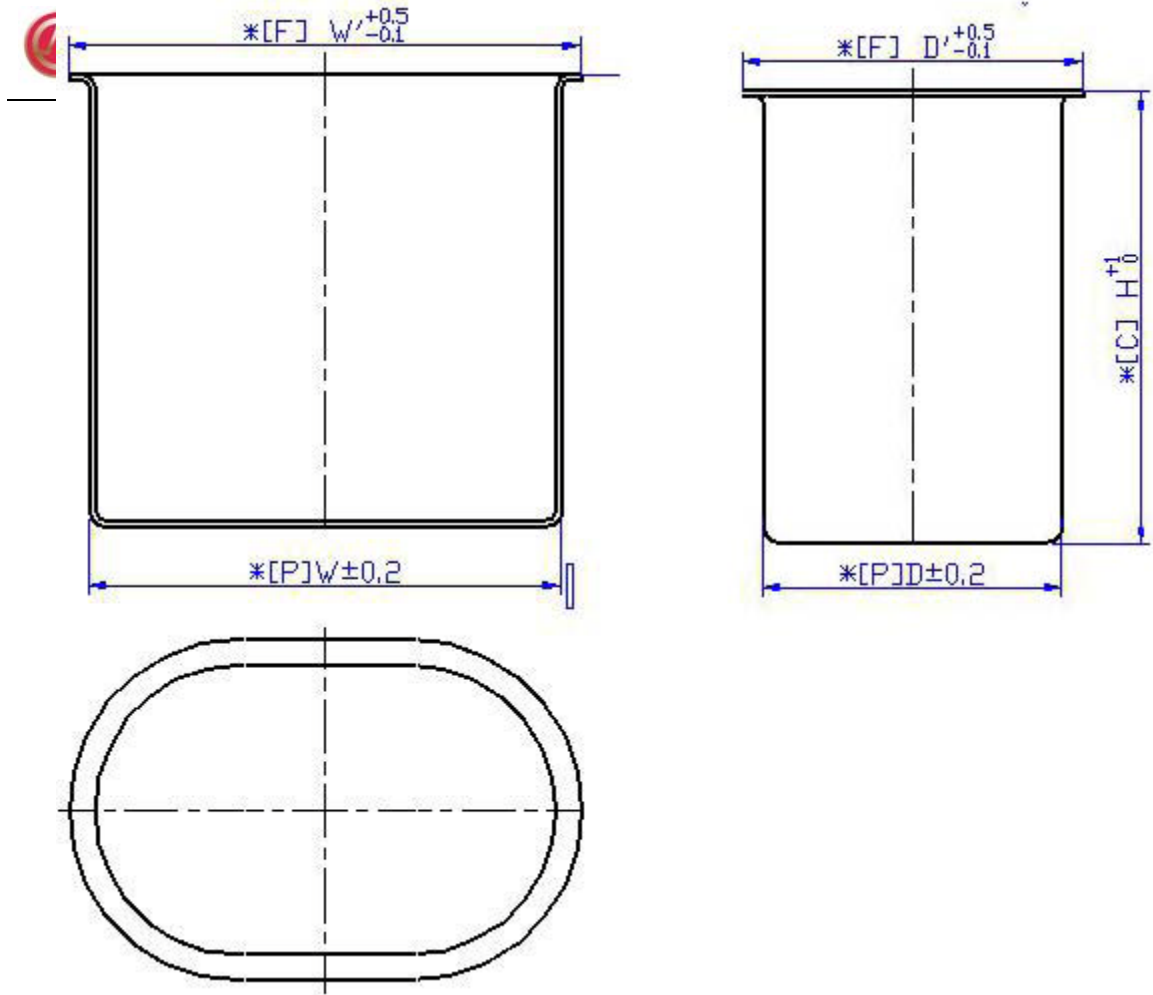
椭圆铝壳
